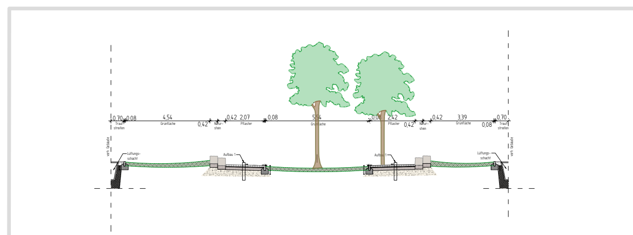
Innenhof II M. 1:200
