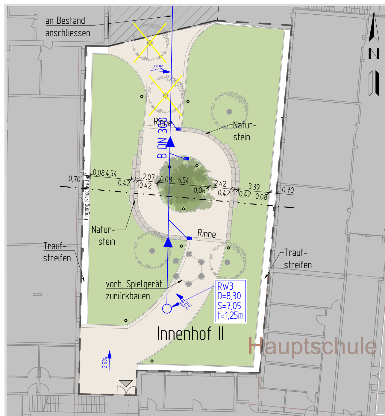
Innenhof II M. 1:250
