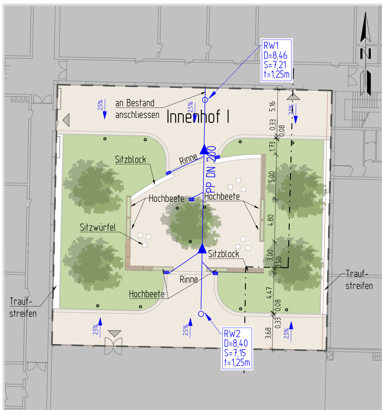
Innenhof I M. 1:250
