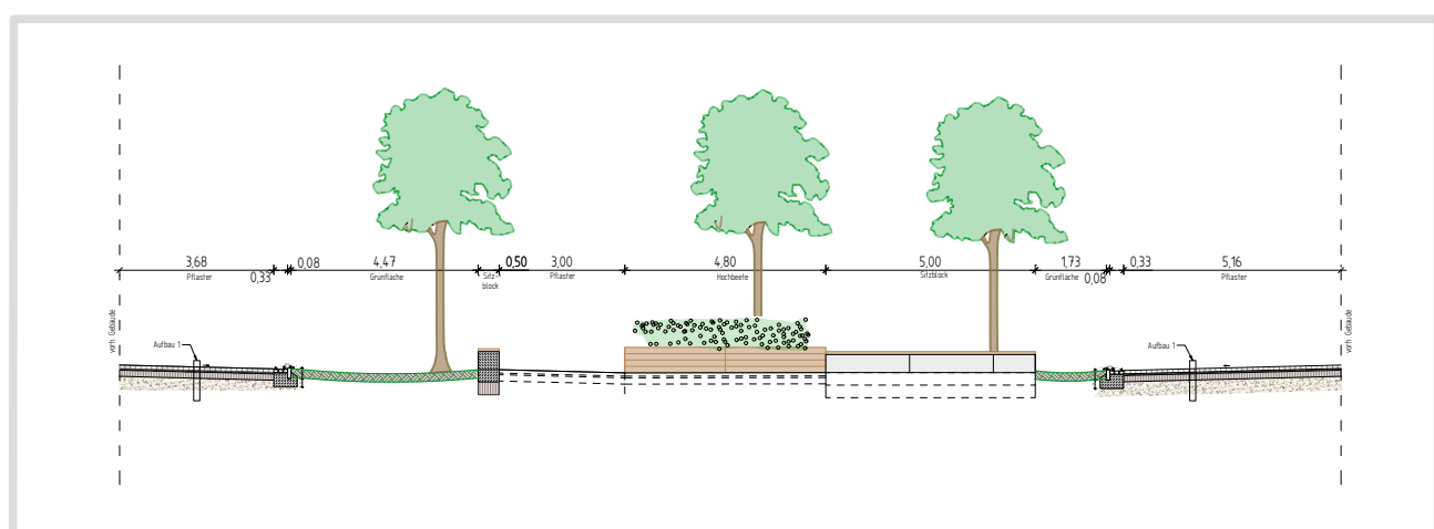
Innenhof I M. 1:200
