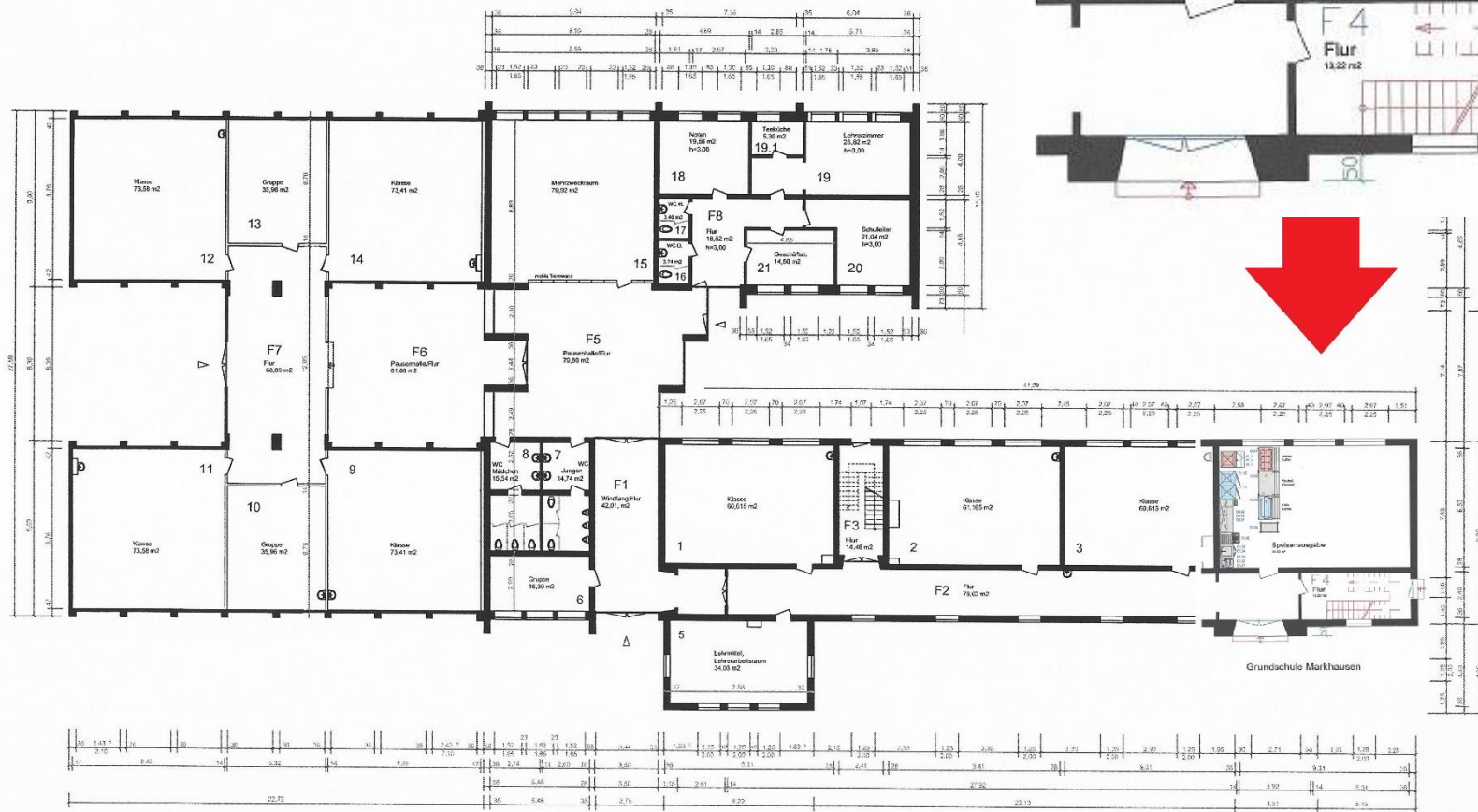
Grundschule Markhausen Erdgeschoss M. 1:200
