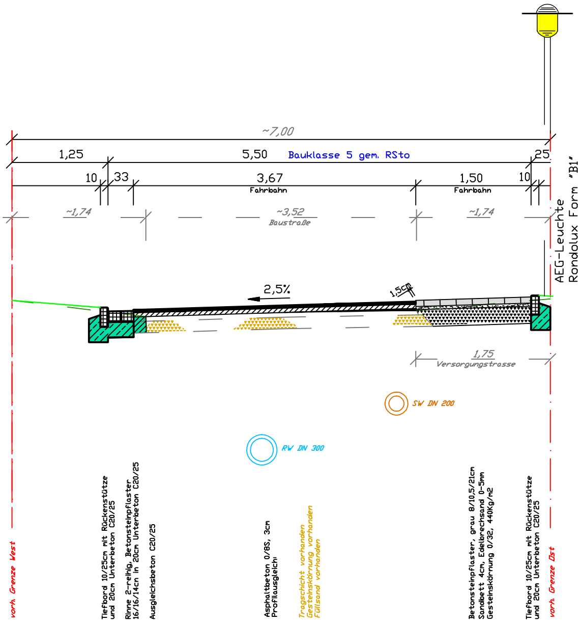
Fuchsweg, M. 1:50
