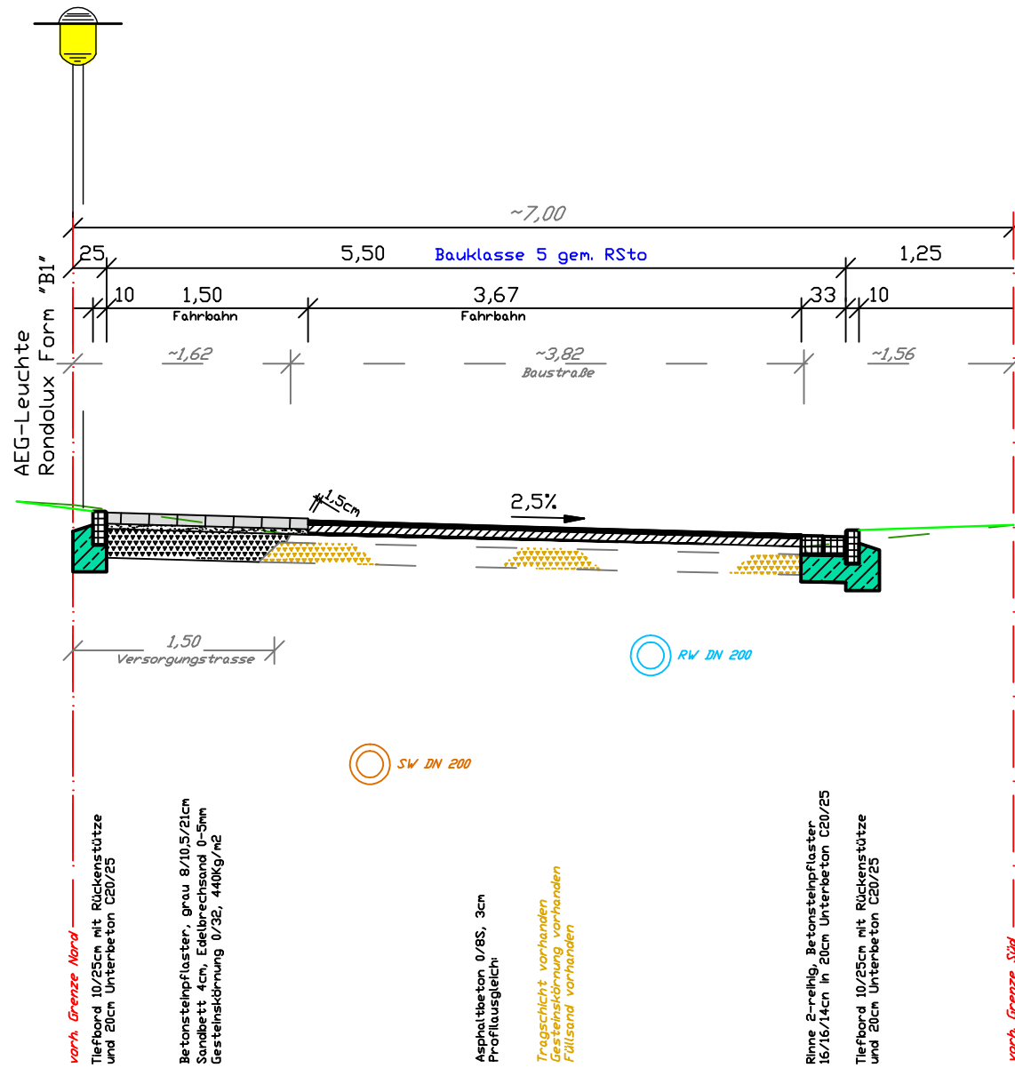
Lautzstraße, M. 1:50
